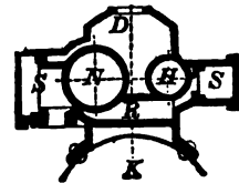
Фиг. 2. Цилиндры и колпакъ большаго Л. компаунда (разрѣзъ) сист. Вольфа.
